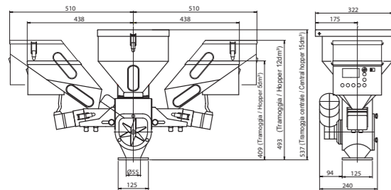
UNITA' DI DOSAGGIO LDM CON MIXER DINAMICO MX3 UNIT DOSING LDM WITH DINAMIC MIXER MX3
